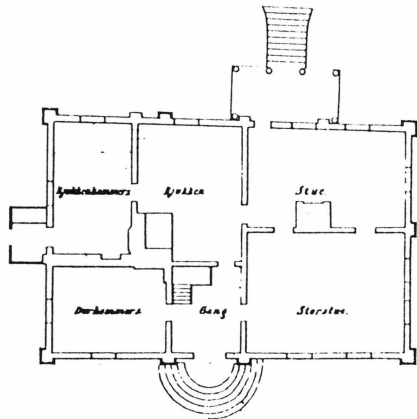
1. Etage.
